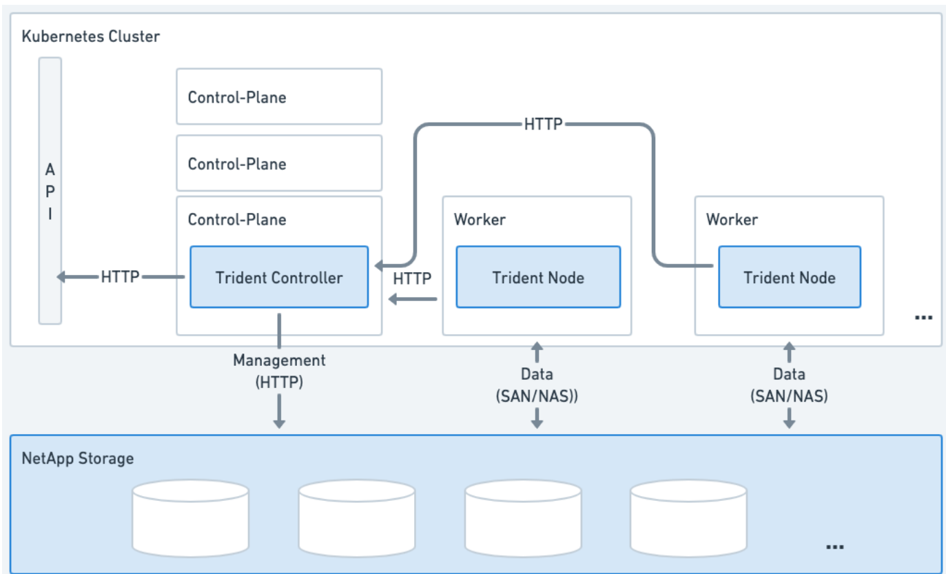
Abbildung 1. Auf dem Kubernetes-Cluster implementierte Trident
