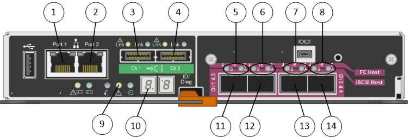
Vista trasera de la controladora E5600SG
