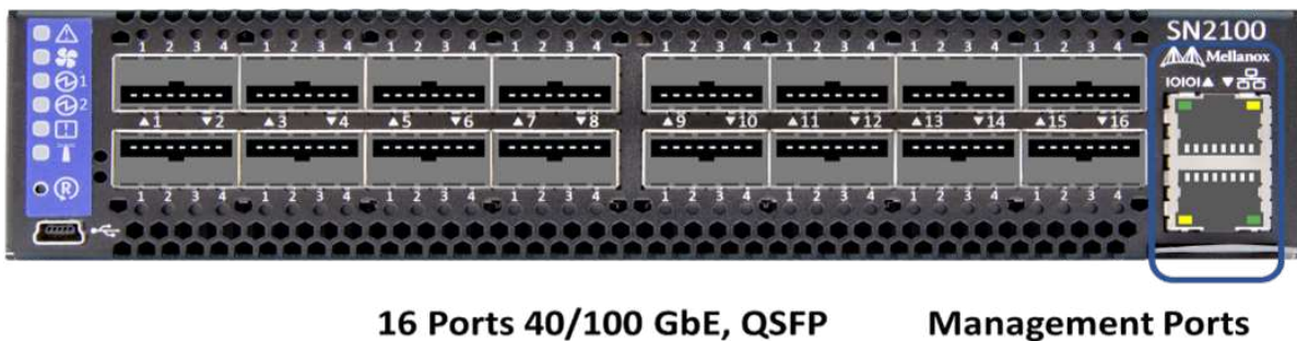
Figure 2. Face avant et ports du commutateur SN2100
