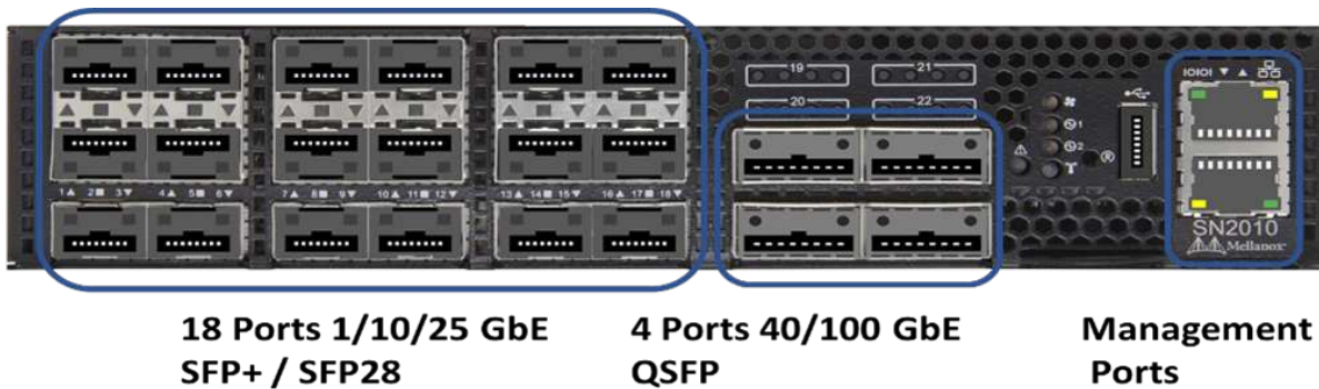
Figura 1. Porta e mascherina dello switch SN2010
