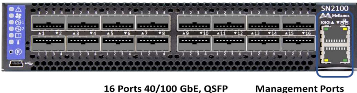
Figura 2. Porta e mascherina dello switch SN2100
