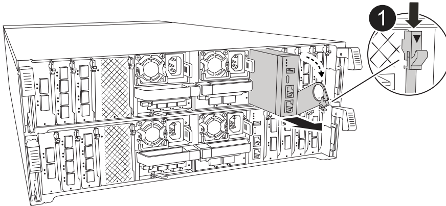
システム管理モジュールのカムラッチ
