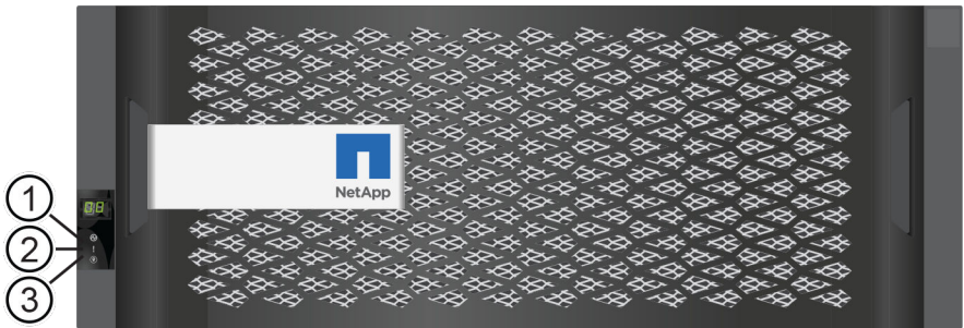
E5760 controller shelf front bezel
