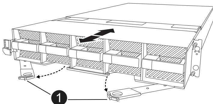
1 Travas do came de travamento
