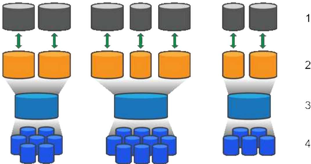
1主机LUN；2卷；3卷组或池；4 HDD或SSD驱动器
