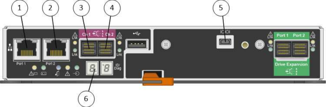
E2700控制器背面图
