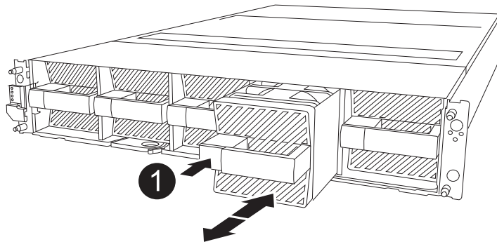
黑色釋放按鈕
