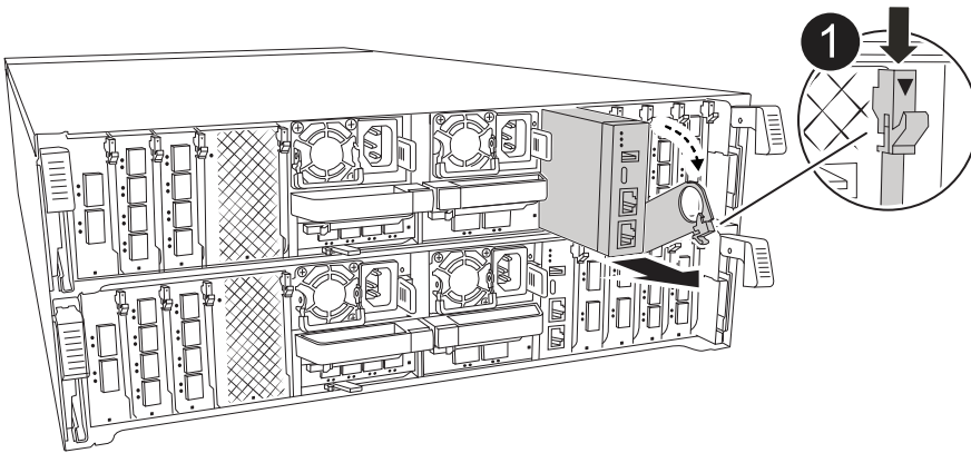
系統管理模組 CAM 栓鎖
